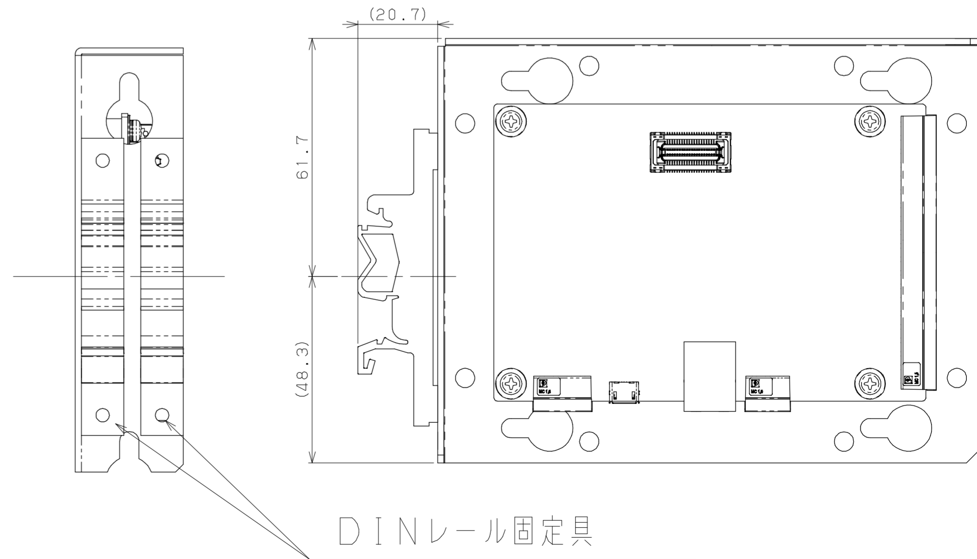
取付例④
