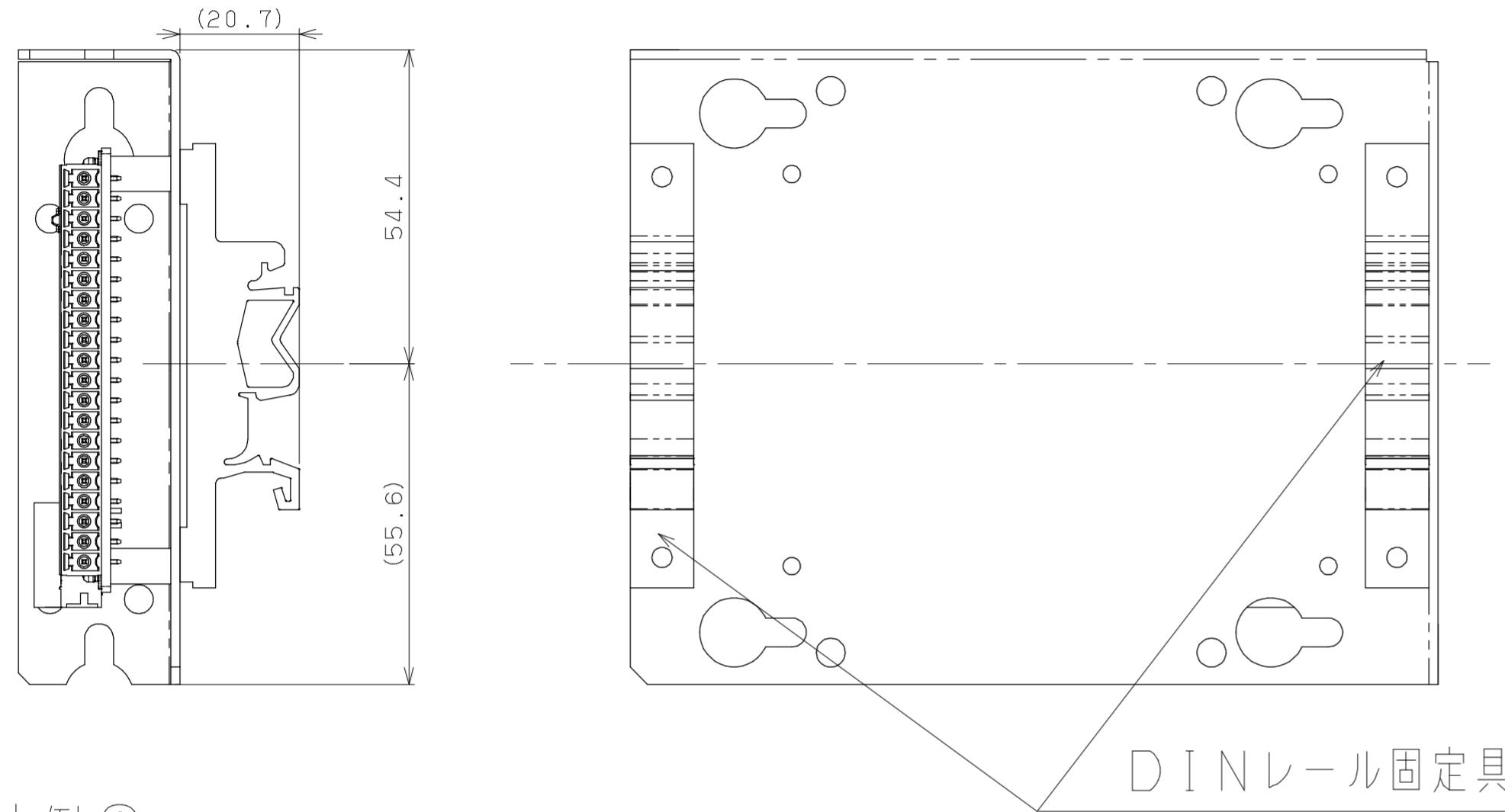
取付例②
