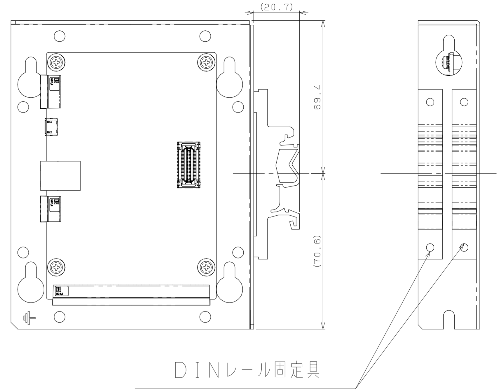
取付例④
