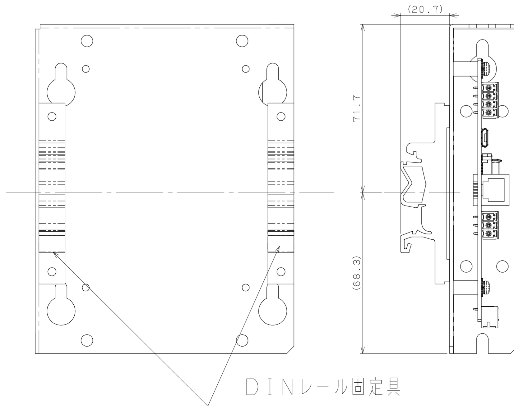
取付例②
