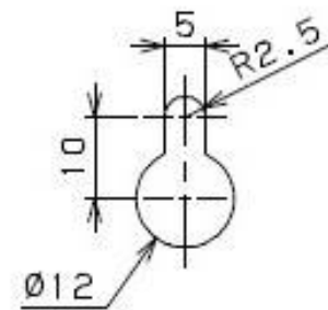
ダルマ穴寸法図
