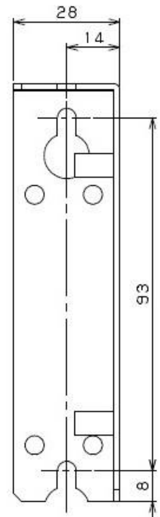
ダルマ穴寸法図
