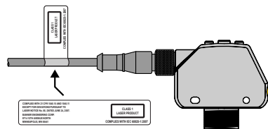
図 3 : 安全ラベルの貼付
