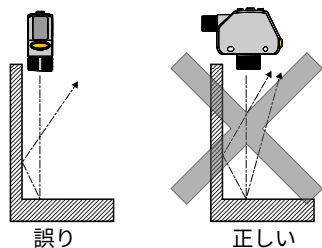
図 5 : 壁際での向き
