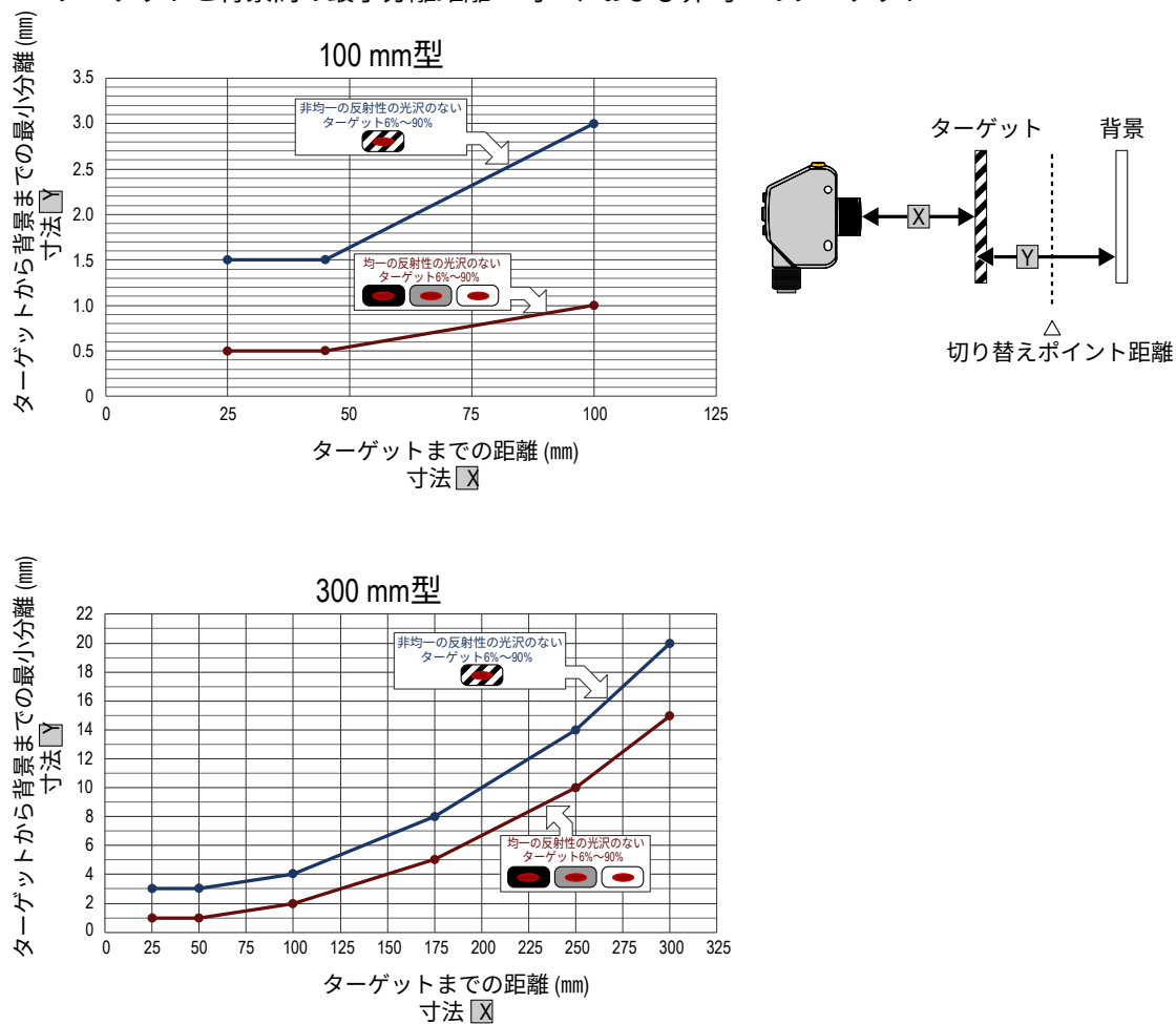
図 17 : 最小対象物分離距離 (90% ~ 6% 反射率)
