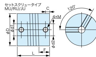
金属製カップリング
