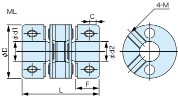
板バネ製カップリング
